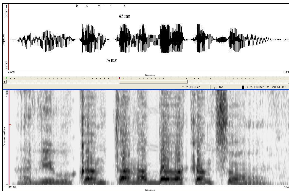
Figura 13: Spettrogramma e forma d'onda dell'enunciato "Avete cantato una bella canzone" prodotta dal soggetto MP (M).
