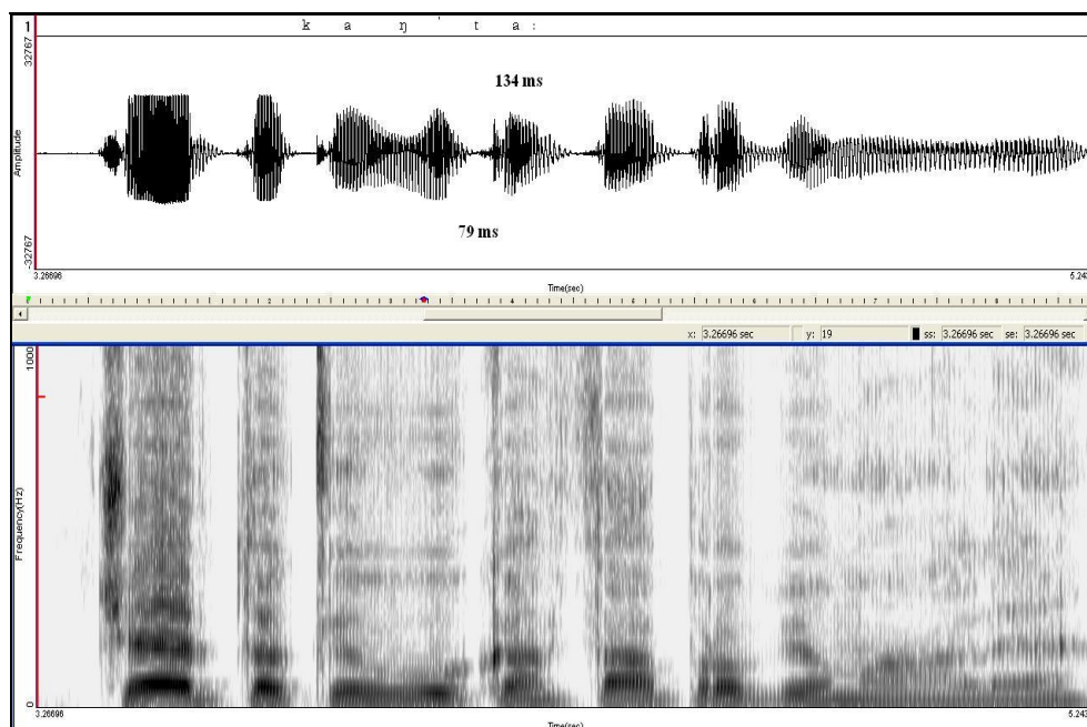
Figura 14: Spetrogramma e forma d'onda dell'enunciato "Certo che voi cantate proprio male" prodotta dal soggetto MP (M).
